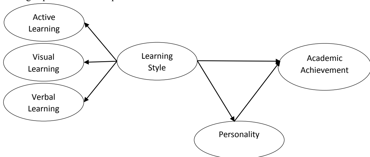
Gambar 1. Kerangka Pemikiran
