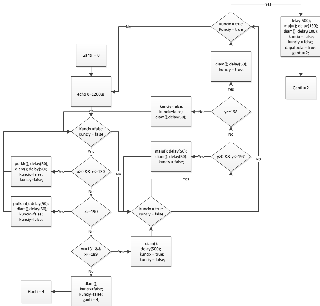
■ Gambar 8. Flowchart Ganti = 0
