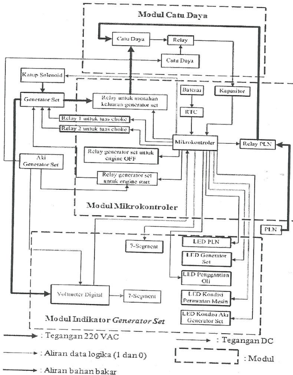
■ Gambar 5. Diagram Blok Alat yang Akan Dirancang
