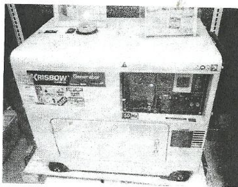
■ Gambar 2. Generator Set Berbahan Bakar Solar Tanpa Fasilitas ATS
