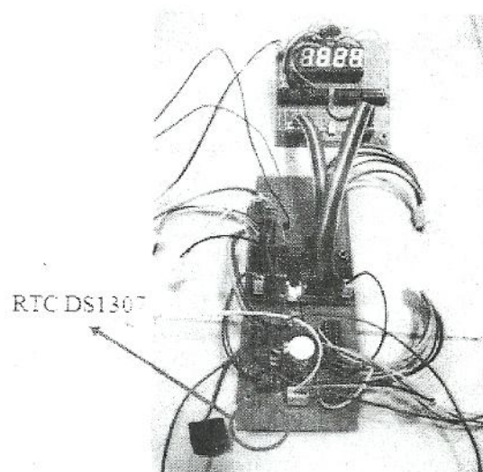
■ Gambar 9. Hasil Pengujian RTC DS1307 Ketika Baru Dinyalakan
