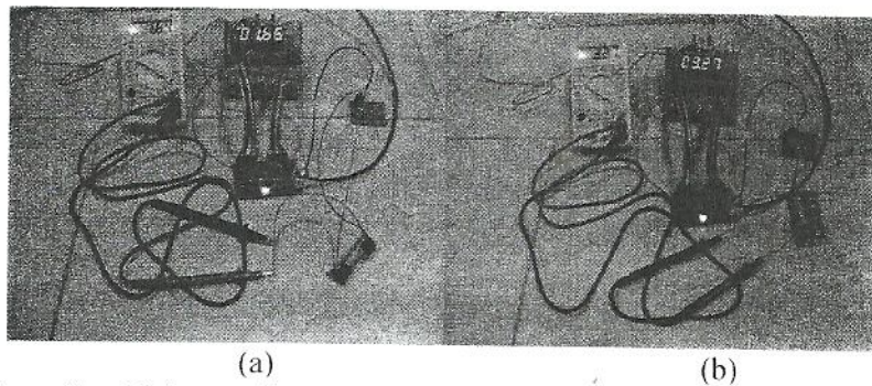
■ Gambar 11. Hasil Pengujian Voltmeter Dengan Satu Baterai 1.5 Volt (a) dan Dengan Dua Baterai 1.5 Volt (b)
