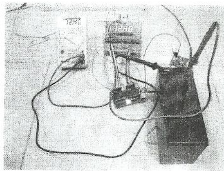
■ Gambar 13. Hasil Pengujian Voltmeter Dengan Aki 12 Volt
