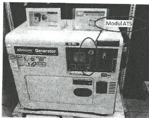
■ Gambar 1. Generator Set Berbahan Bakar Solar dengan Fasilitas ATS
