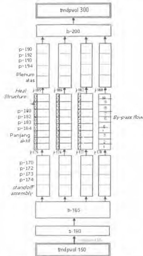
Gambar 4. Nodalisasi model perangkat bahan bakar
