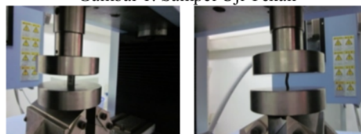
Gambar 2. Proses Uji Tekan
